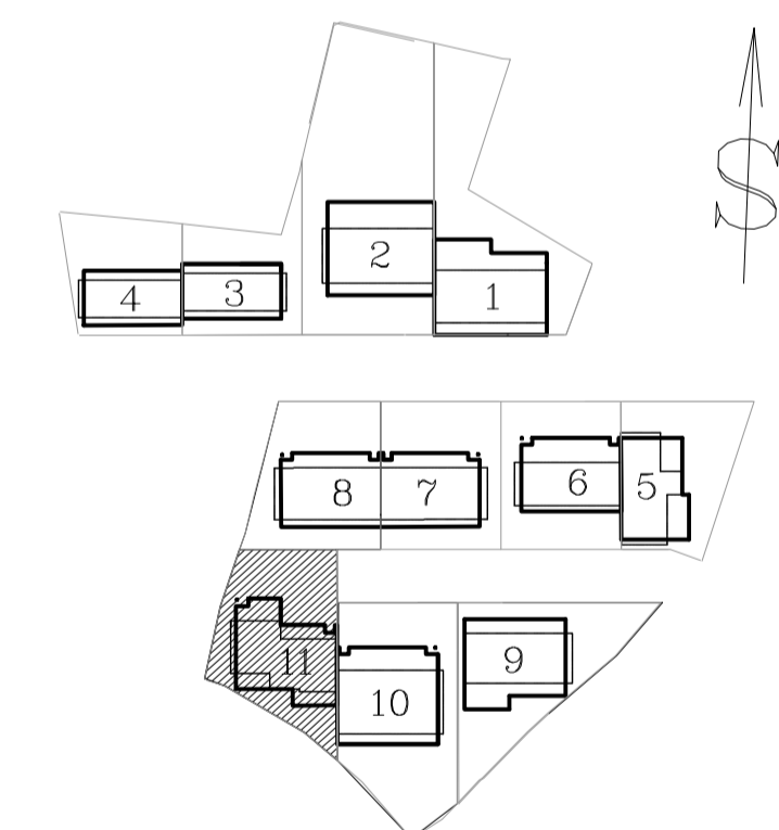
situacija objekat 11
