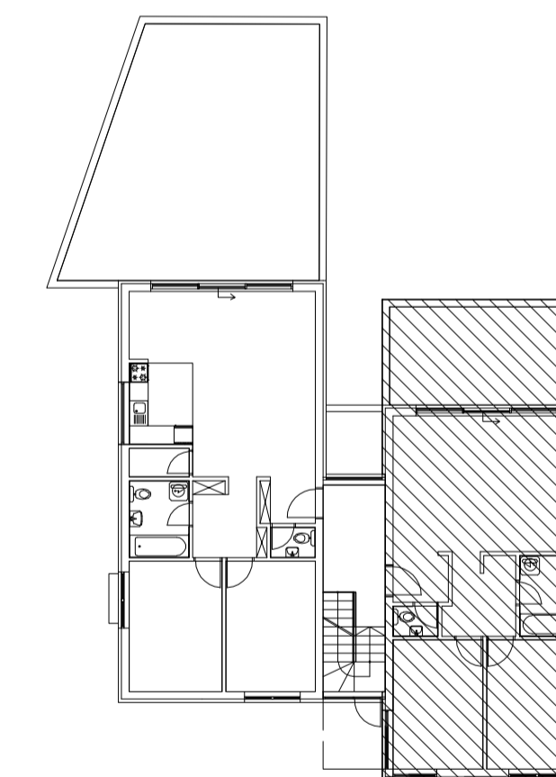
prizemlje
